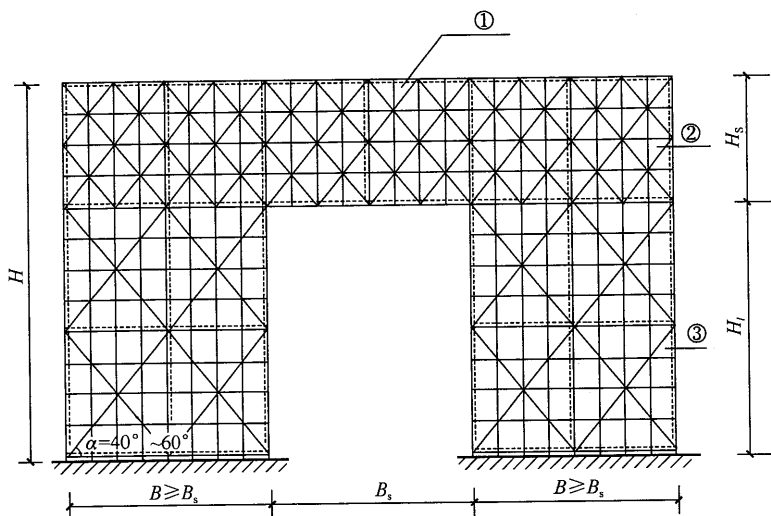
(a) 立面图
