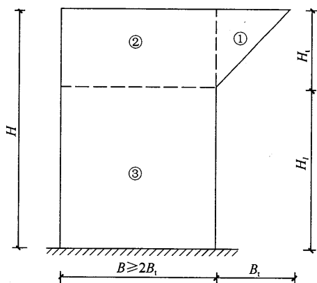
图 15 悬挑支撑结构分区图
