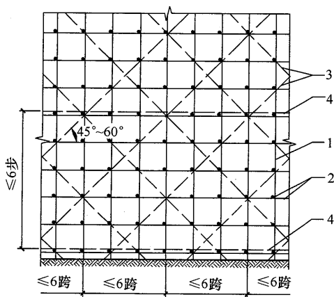
(b) 立面图
