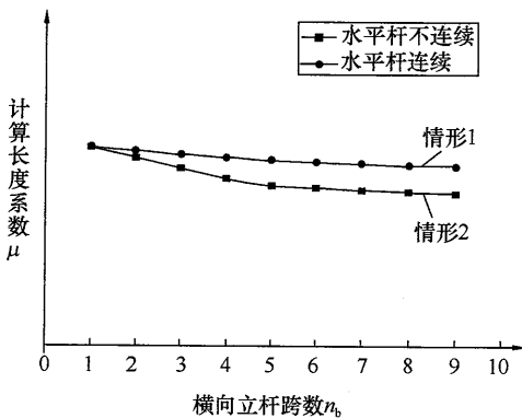
图 12 无剪刀撑框架式支撑结构 \mu 随立杆横向跨数 n_b 变化示意图
