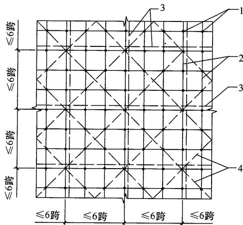
(a) 平面图
