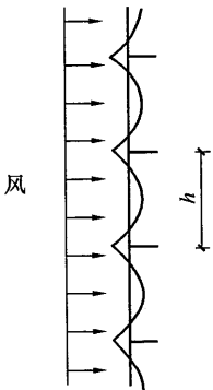
图 10 立杆节间局部弯矩立面图
