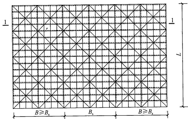
(b) 平面图
