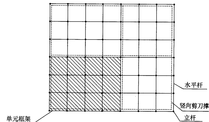
图 1 单元框架平面示意图
