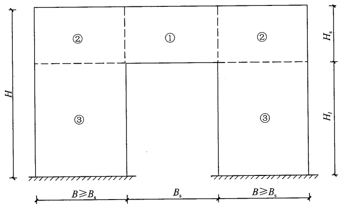
图 16 跨空支撑结构分区图
