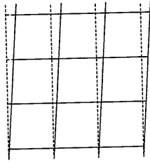
图 2 无剪刀撑框架式支撑结构的失稳模态图
