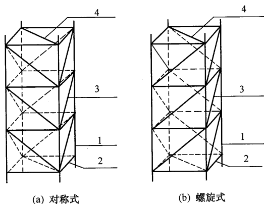
图 5.3.1 单元桁架斜杆布置立面图
