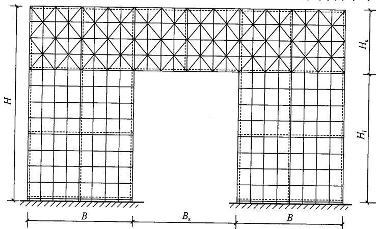
图 6.2.3 跨空支撑结构剖面图 (1-1)
