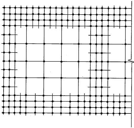
图 5.2.7 支撑结构不同立杆间距布置平面图
