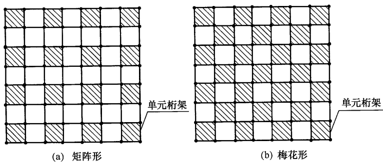
图 5.3.2 单元桁架组合方式布置平面图
