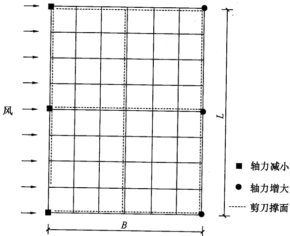
图 4 风荷载作用于有剪刀撑框架式支撑结构引起的立杆轴力图（俯视图）
