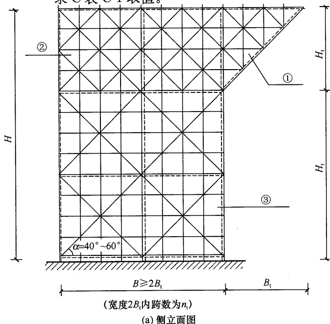
图 6.1.1 悬挑支撑结构示意图 (一) ①—悬挑部分; ②—平衡段; ③—落地部分 注: 虚线表示垂直于图面的剪刀撑或斜杆。
