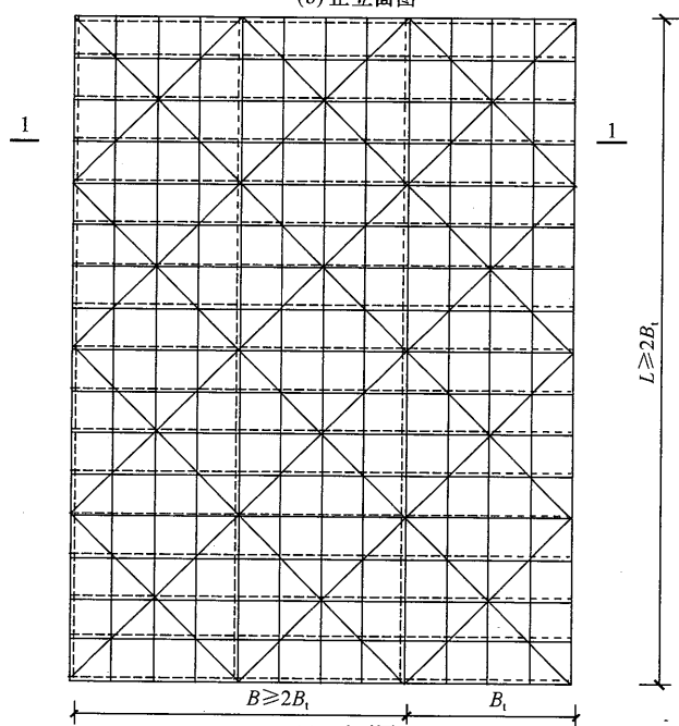
(c) 平面图
