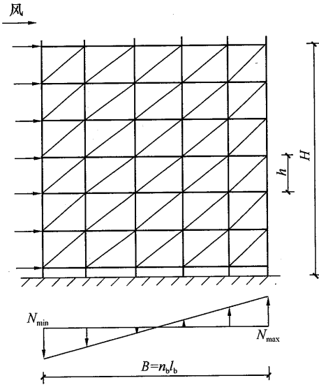
图 9 桁架式支撑结构（梅花形）风荷载引起的立杆轴力图
